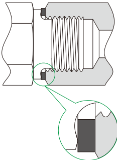
2.GB阳螺纹，根部垫片和FG阴螺纹
